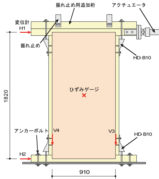
面材釘試験体
