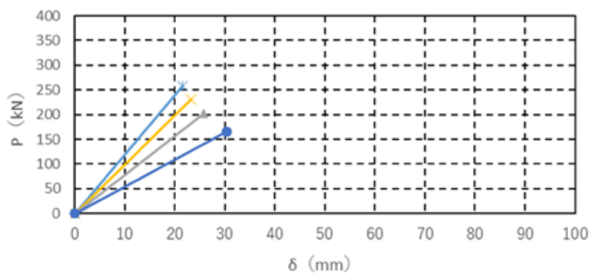
構面高さ 3.5m の荷重変形関係の計算値
