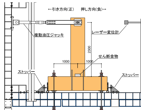
加力装置 (単位: mm)
