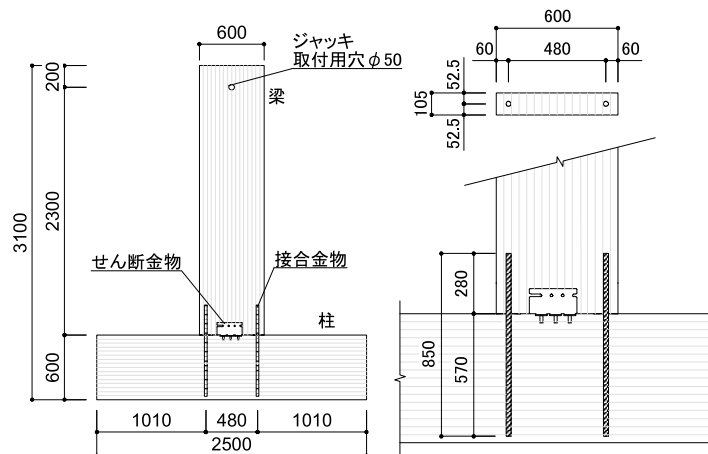
G-TM 試験体図 (単位: mm)
