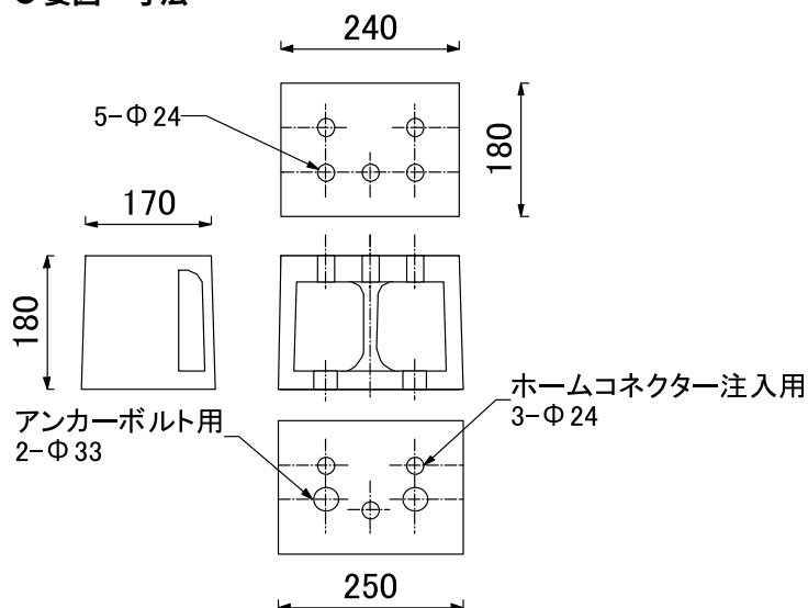
柱脚金物(240 × 180)詳細図(単位:mm)
