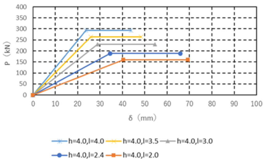
構面高さ 4.0m の荷重変形関係の計算値
