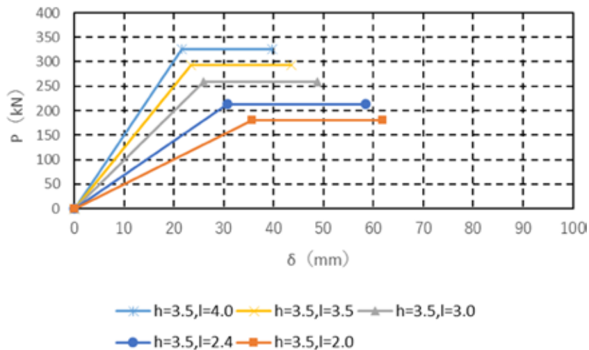
構面高さ 3.5m の荷重変形関係の計算値
