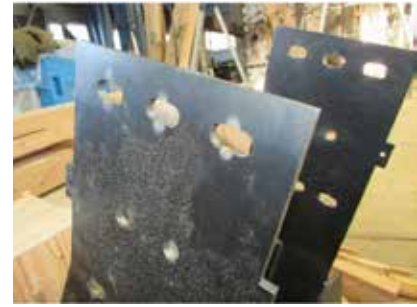
解体後 PL 支圧変形
