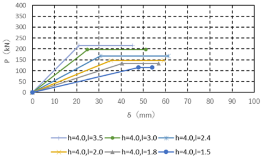
構面高さ 4.0m の荷重変形関係の計算値 (上：正側加力、下：負側加力)
