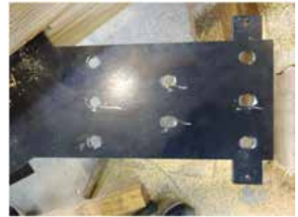
鋼板の支圧変形
