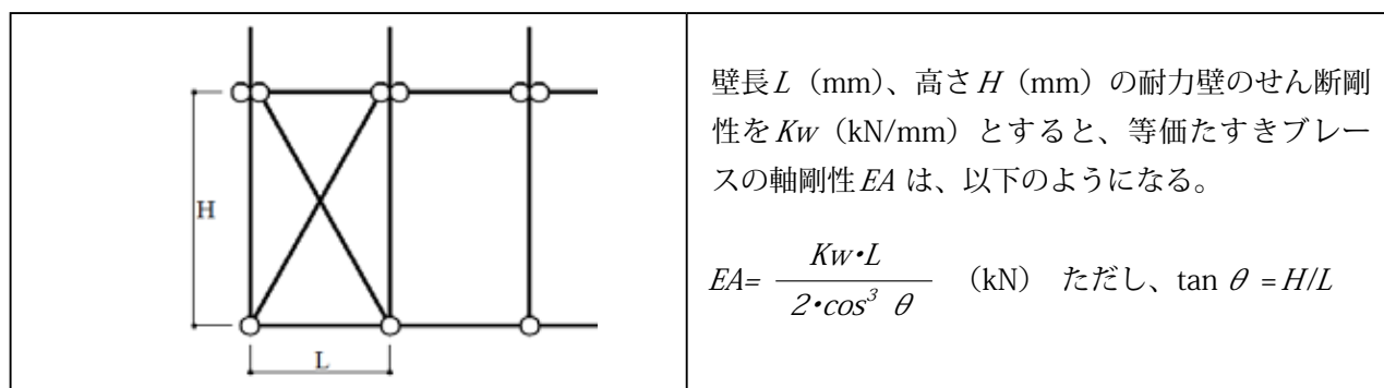
面材張り耐力壁のモデル化
