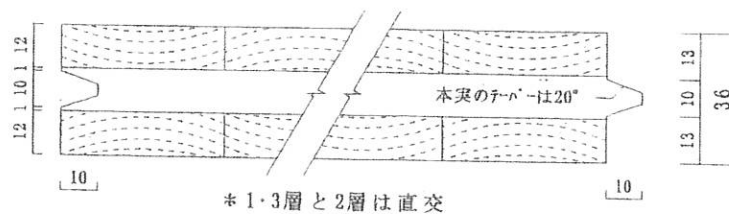
図1 断面形状図
