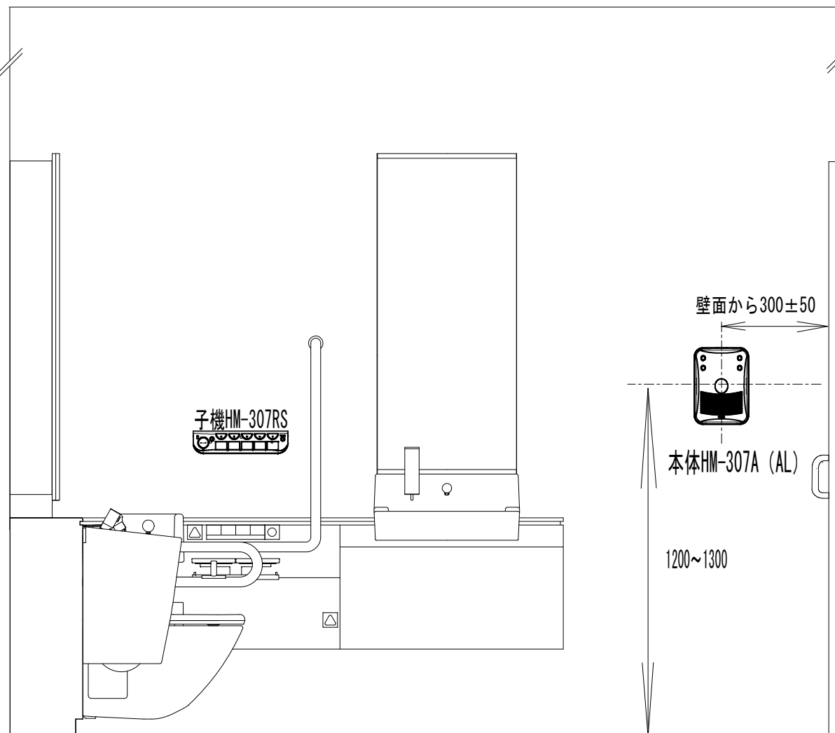
【展開図】
