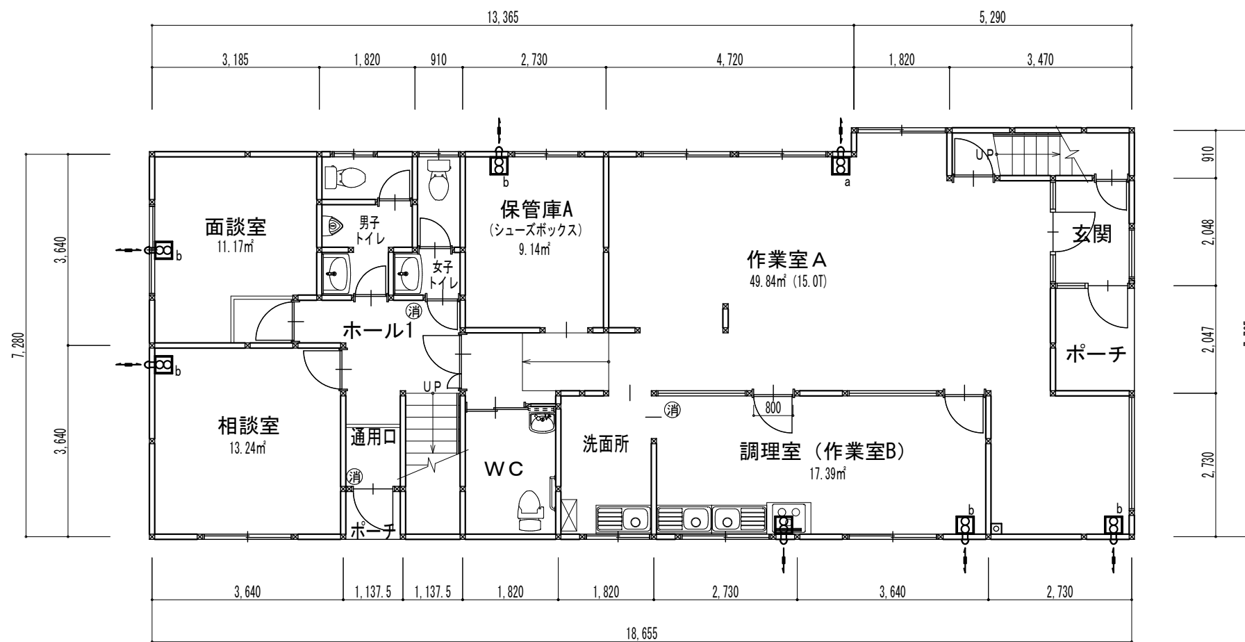
1階平面図
