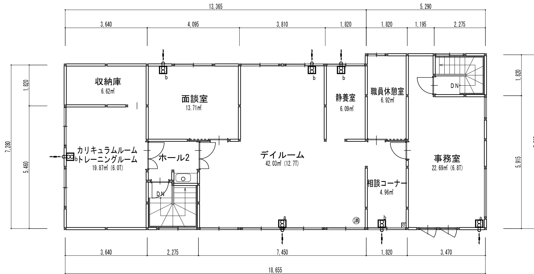
2階平面図
